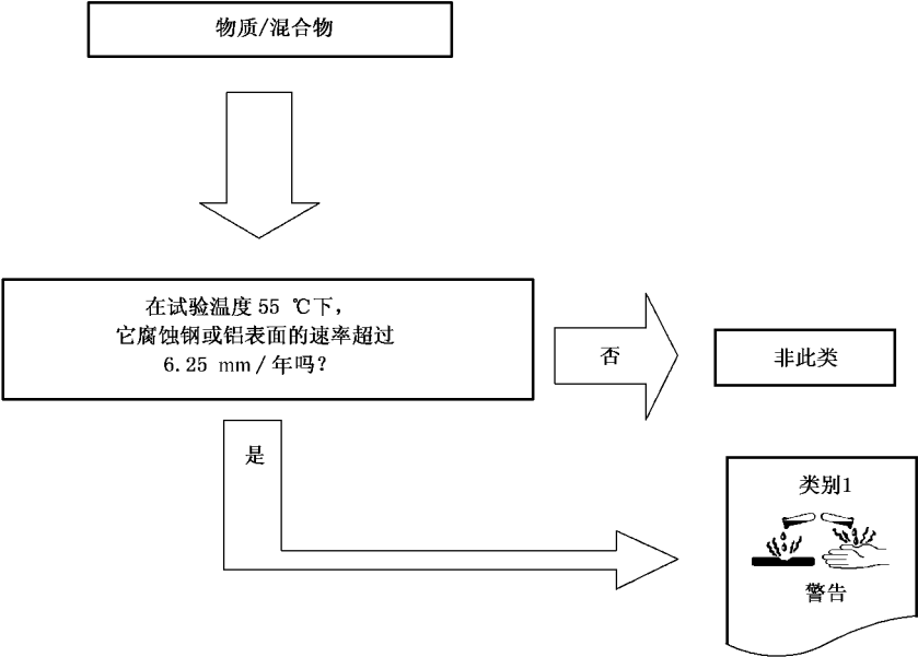
图 A.1 金属腐蚀物的判定逻辑
